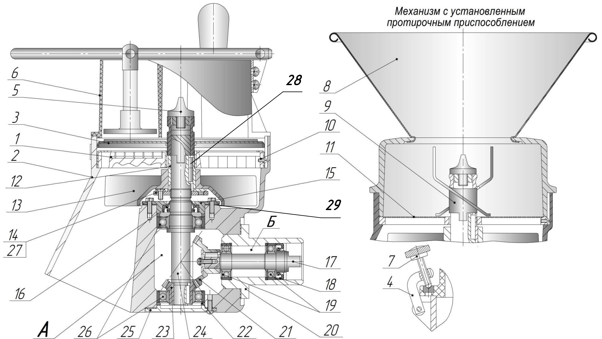
Механизм овощерезательно-протирочный МО
